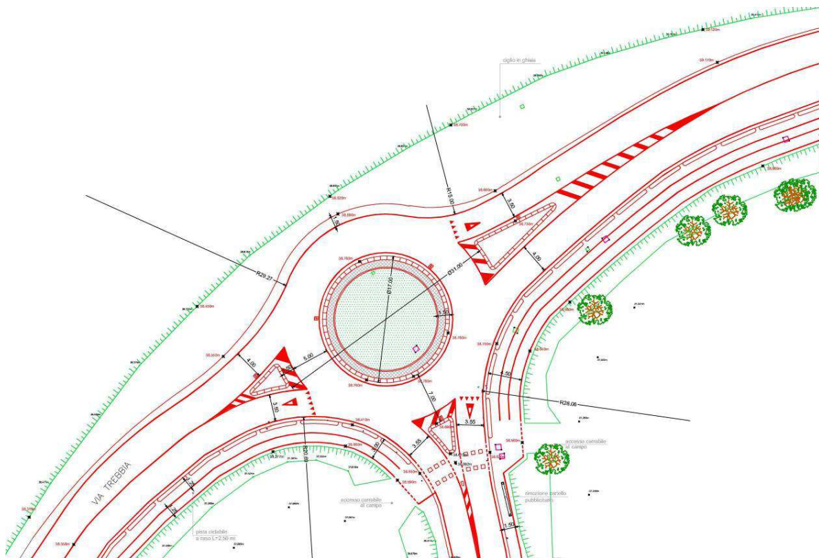
PROGETTO - Zona centrale dell'intervento – rotonda e isole spartitraffico
