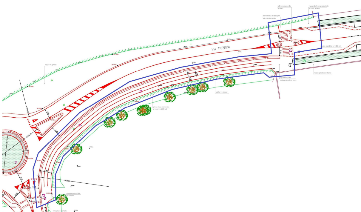
PROGETTO - Zona est dell'intervento – pista ciclopedonale, attraversamento e marciapiede di via Trebbia
