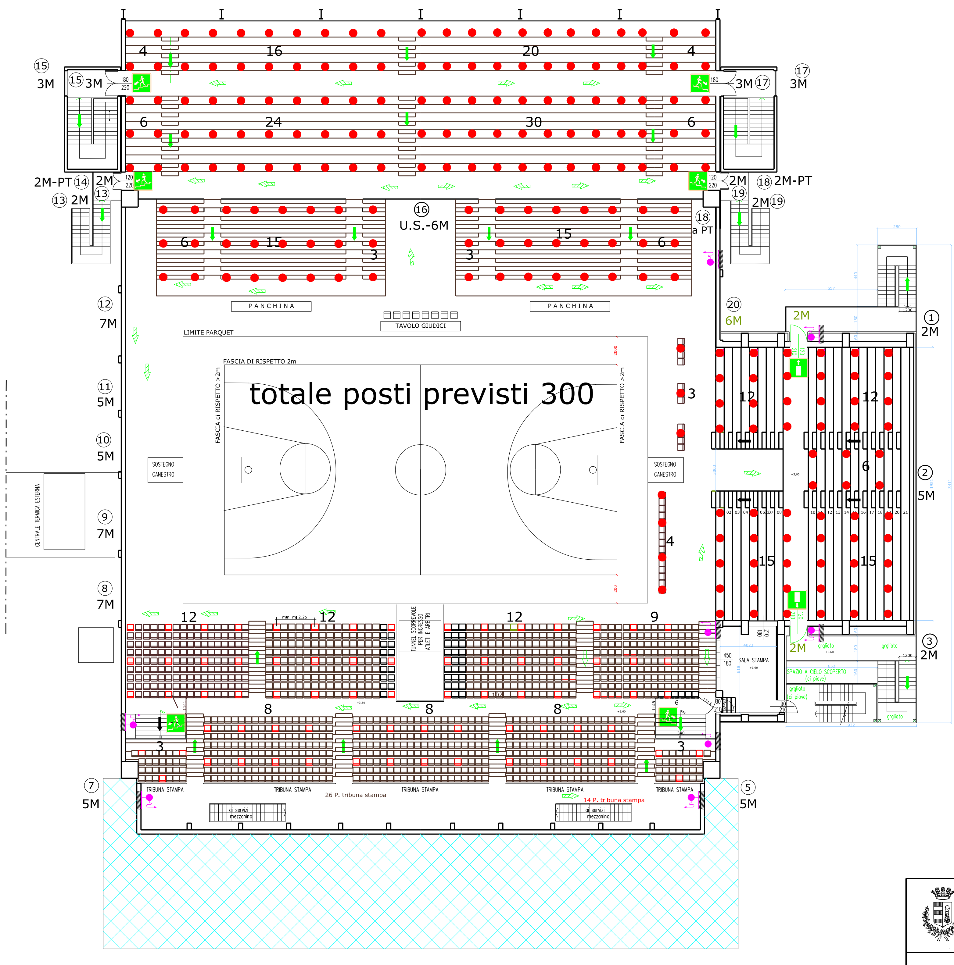
PIANO PRIMO
